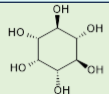
Mioinositol
