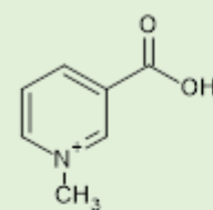
Trigonelina
