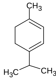
Terpineno
