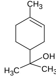
Terpineol
