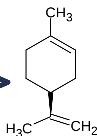
Limoneno
